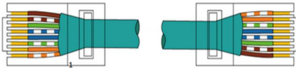
T568B
