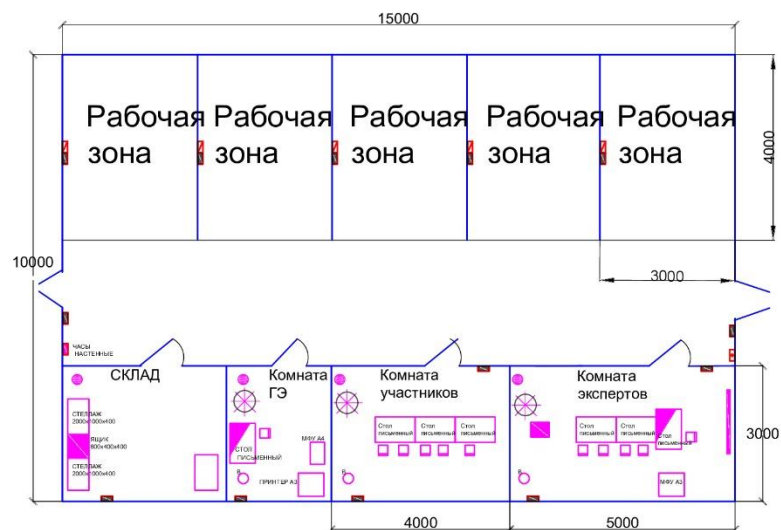
Общий план застройки рабочей площадки
