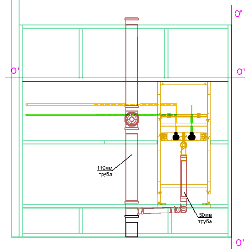
Вид "В"
