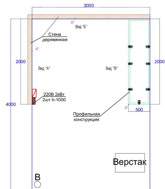
План рабочей зоны
